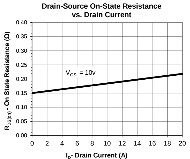
Fig.13 I_D - R_{DS(ON)}
