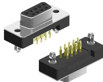
Press Fit Type
