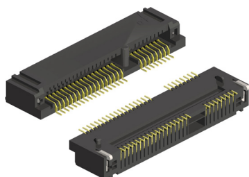
Qseven / MXM Connectors M.2 Mini PCI Express
