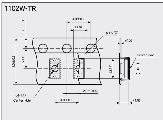
テーピング寸法図／Taping specification
