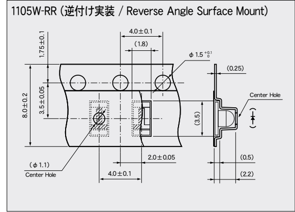
テーピング寸法図／Taping specification (unit : mm)
